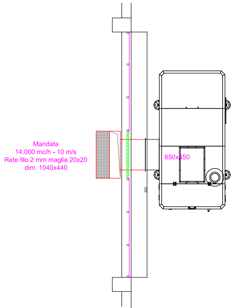
PIANTA MANDATA
