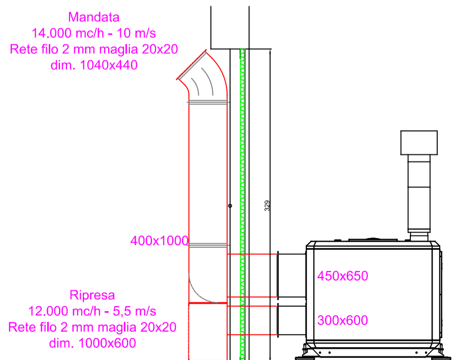
VISTA LATERALE
