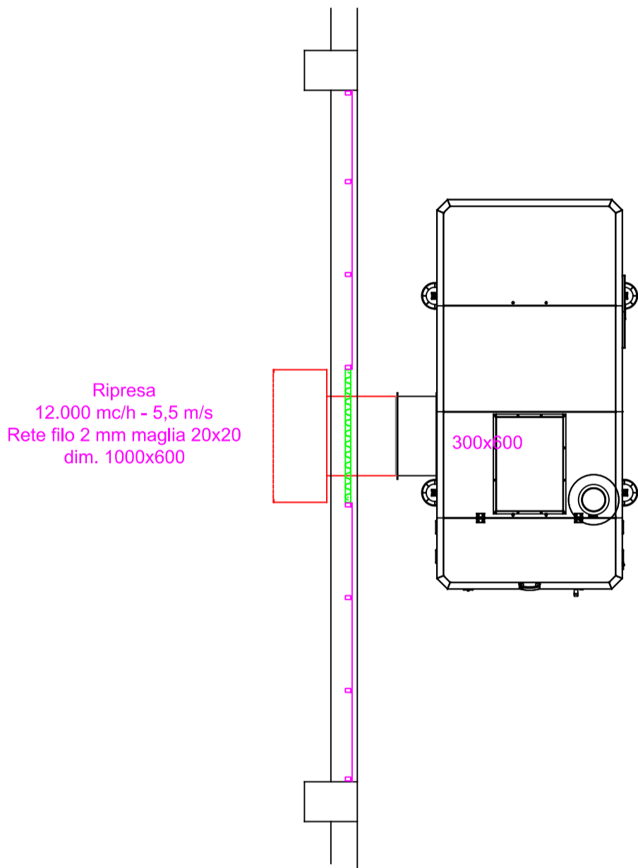
PIANTA RIPRESA
